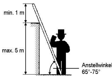
Anstellwinkel und min. Länge für Anlegeleitern
