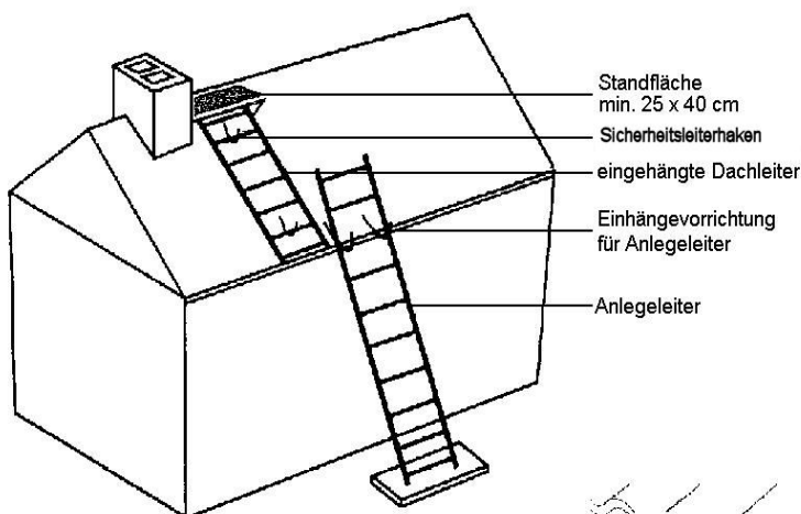
Sicherheitsleiterhaken bzw. Einhängvorrichtung für Dach- und Anlegeleitern
